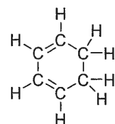
1,3-シクロヘキサジエン
