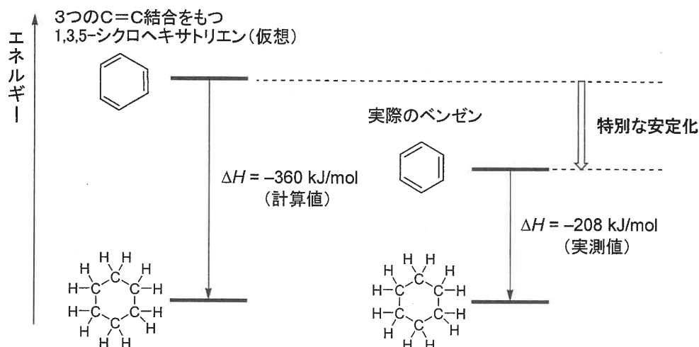
図：ベンゼンの水素化熱の実測値と計算値の比較
